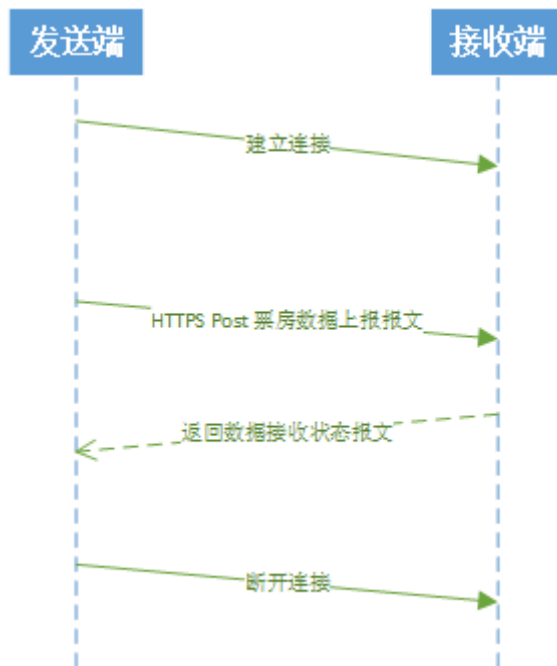
图F.1 票房数据统计上报通信过程
