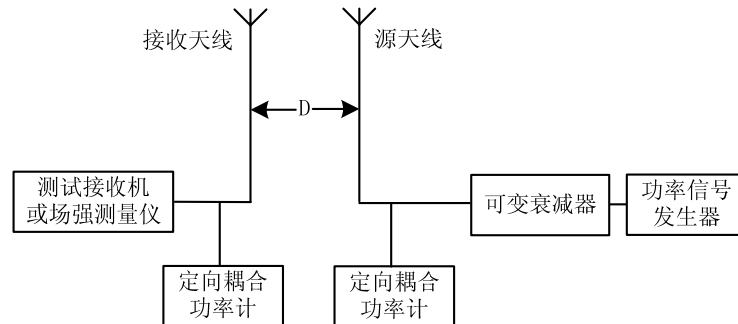
图 4.3.2 增益测量方框图（两相同天线法）
