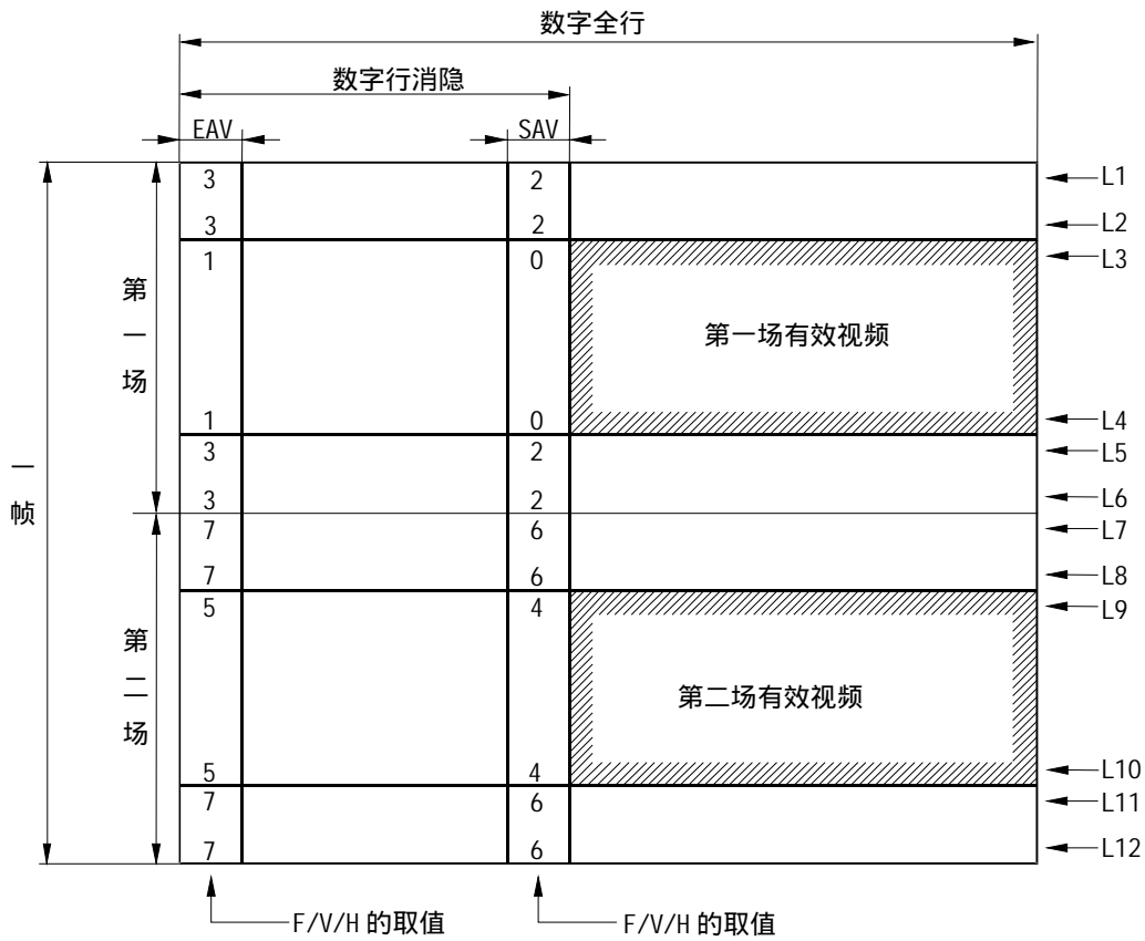
(a) 隔行扫描系统
