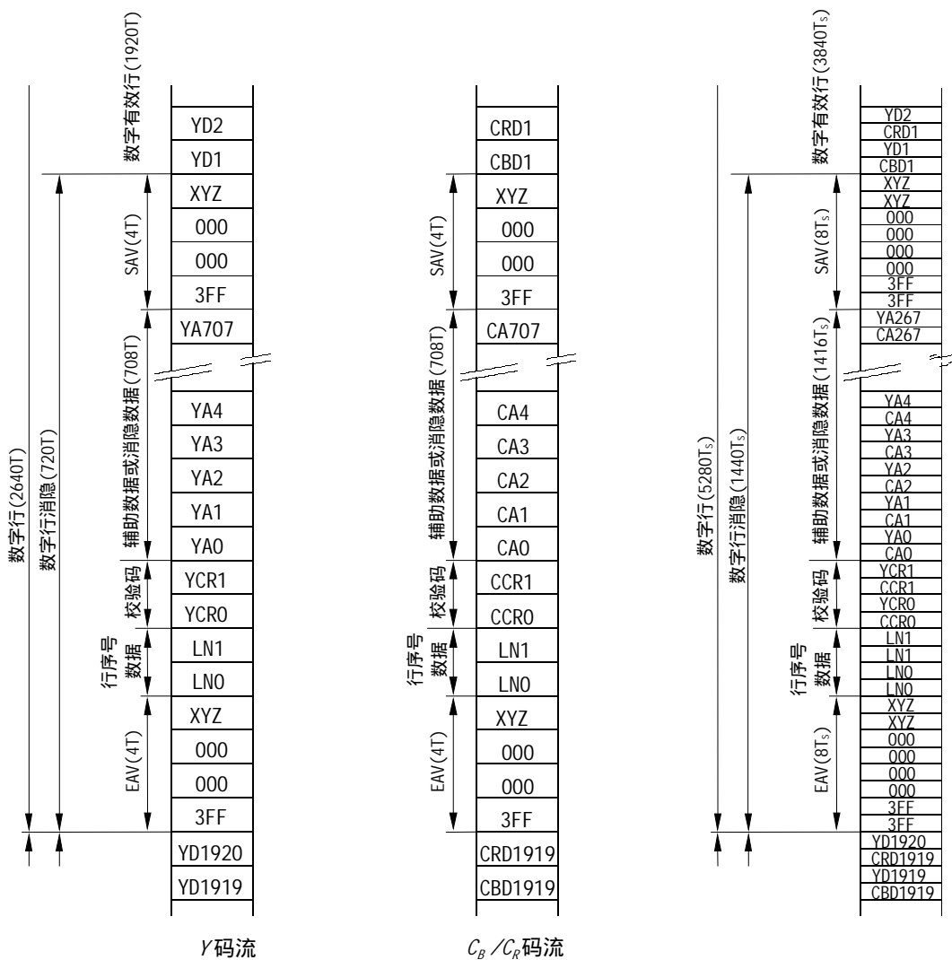
(b) 复用后的并行数据流
