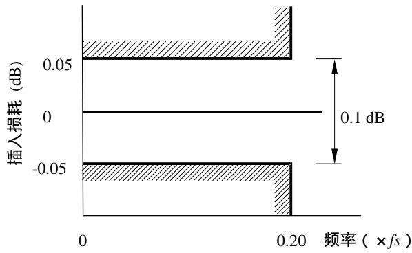
b) 通带起伏容限
