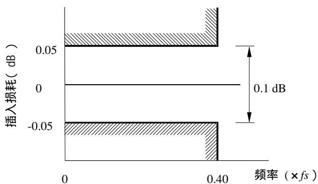
b) 通带起伏容限
