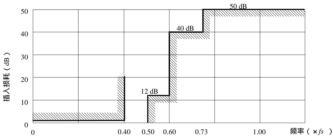
a) 插入损耗特性
