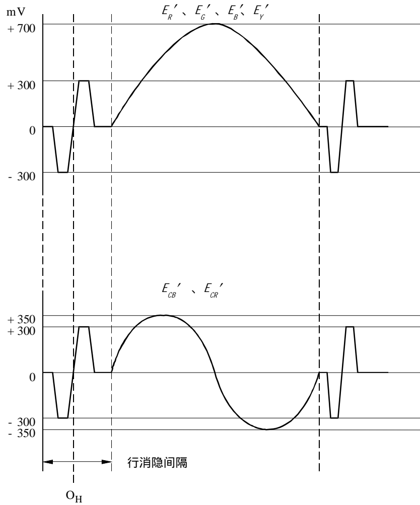
图1 分量信号上的同步电平
