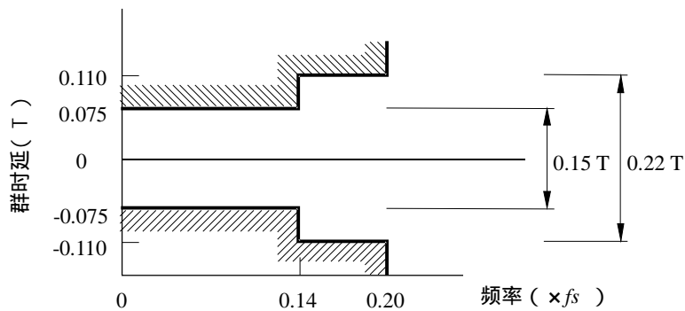
c) 通带群时延
