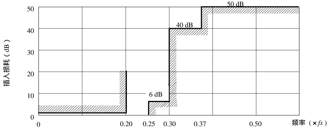
a) 插入损耗特性
