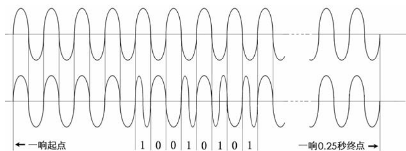
图1 二进制数10010101调制编码的波形
