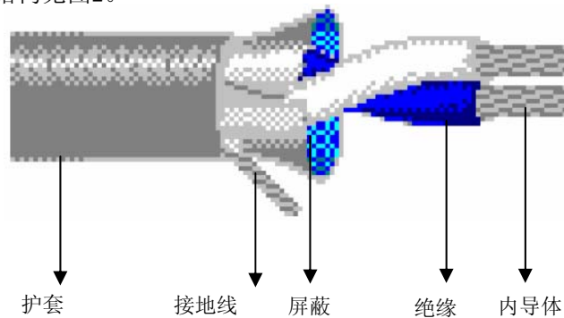
图2 数字音频双绞电缆的结构
